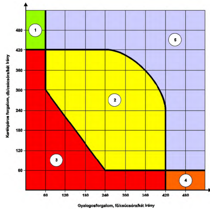
6.2. ábra – A kerékpáros és a gyalogosforgalom szétválasztása
